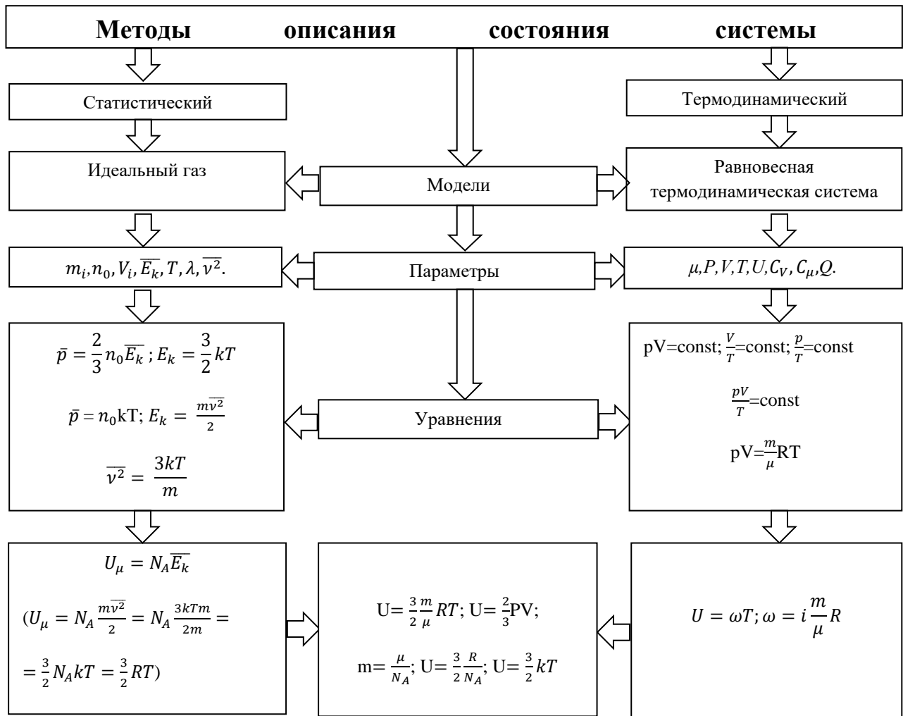
Рис 3. Два метода описания состояния системы
