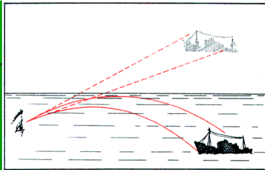
Рис. 10.10. Верхний мираж.
